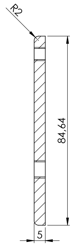
COUPE A-A
