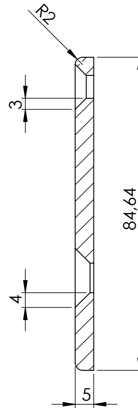
COUPE A-A
